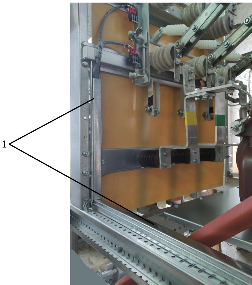
Рис. 10. Кабельные каналы для прокладки жгутов проводников вторичных цепей
