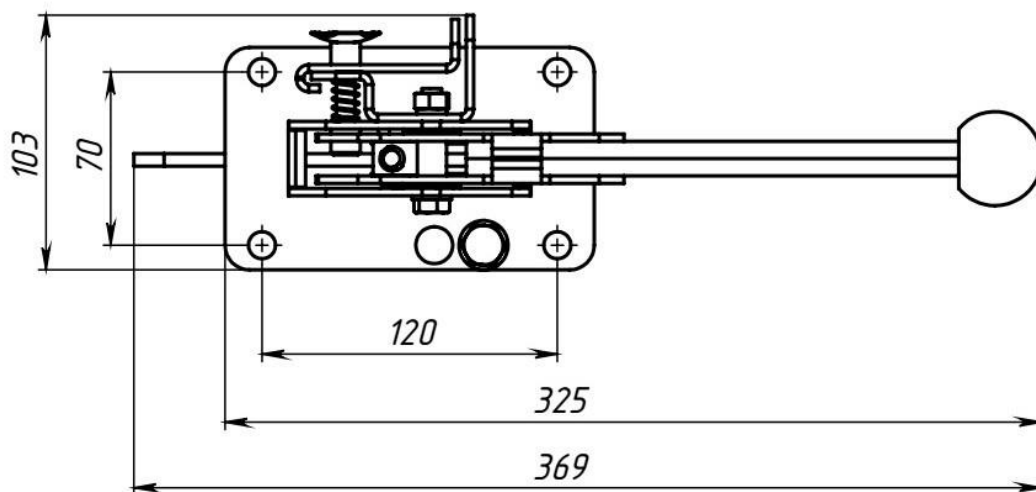
Рис. 6.1. Конструкция привода разъединителя ПР-10
