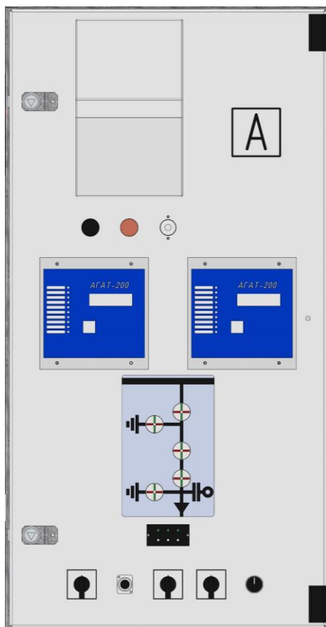
Рис. 3. Дверь модуля вторичных цепей шкафа КСО
