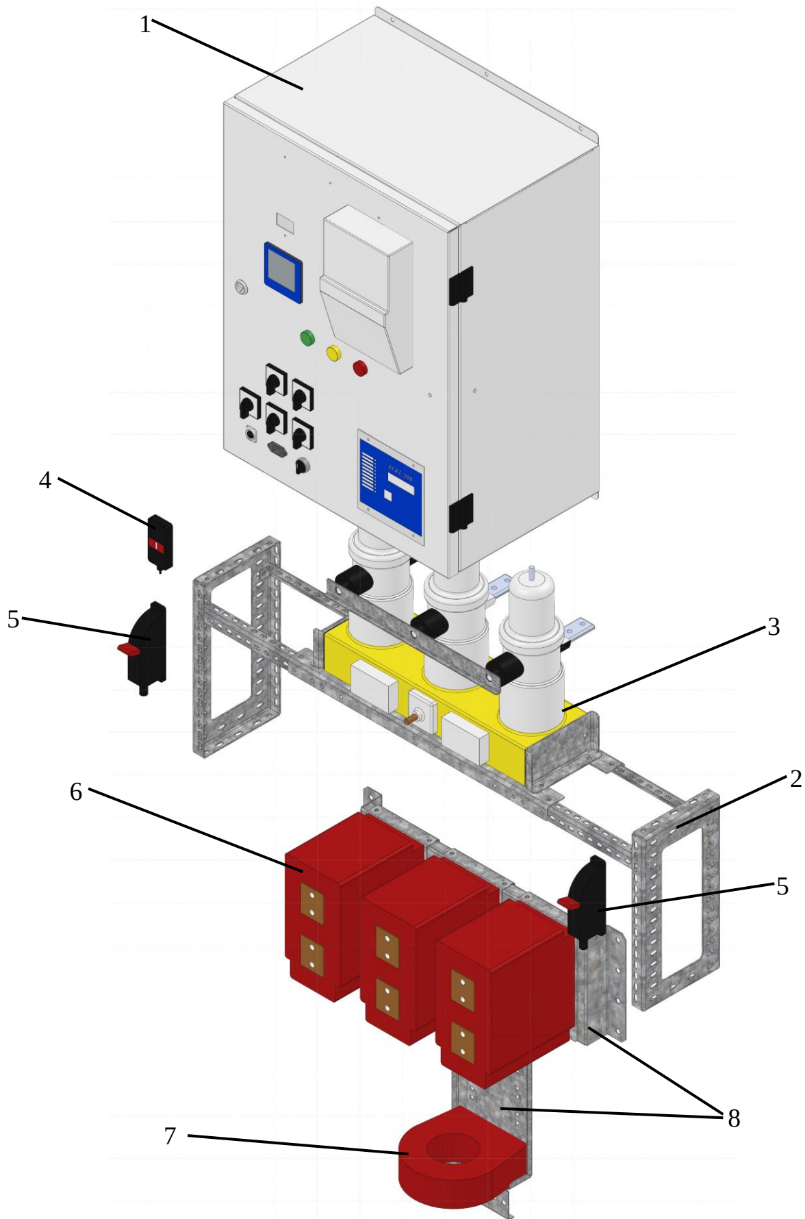
Рис. 1. Основные функциональные элементы комплекта адаптации КСО 1 – релейный модуль; 2 – рама крепления вакуумного выключателя; 3 – вакуумный выключатель; 4 – механический указатель положения вакуумного выключателя; 5 – блокировка разъединителя РВЗ-10 и вакуумного выключателя; 6 – измерительные трансформаторы тока; 7 – измерительный трансформатор тока нулевой последовательности; 8 – каркас установки трансформаторов тока.
