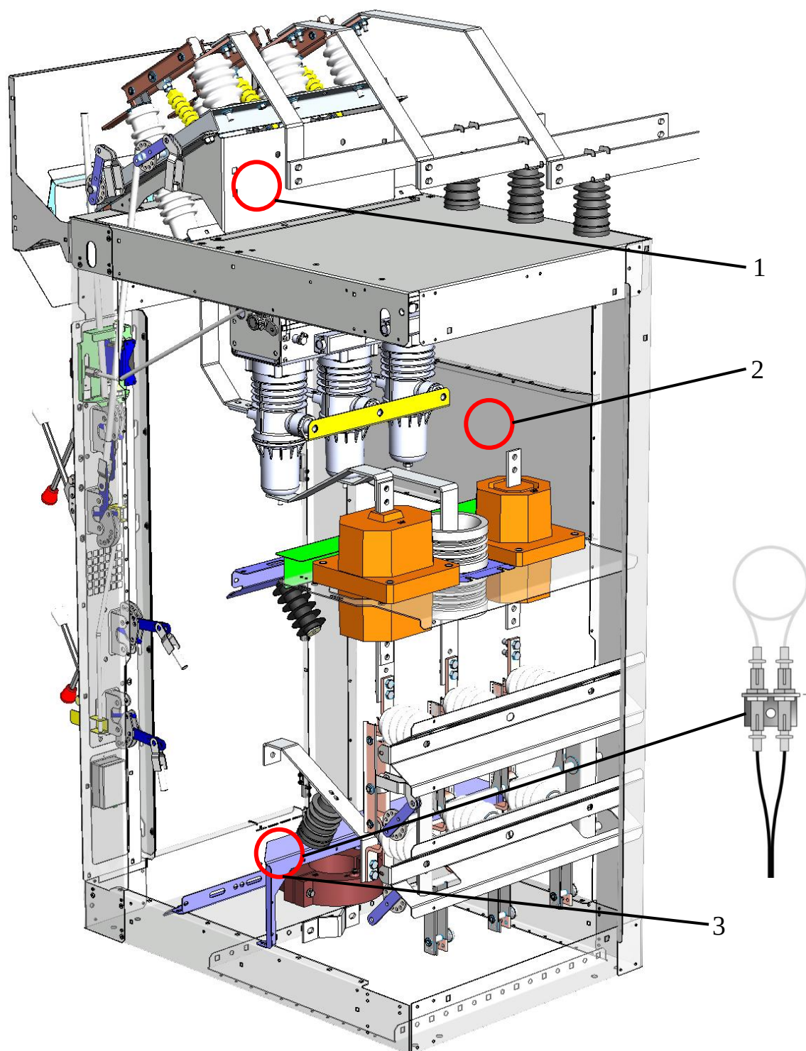
Рис. 9. Места установки датчиков дуговой защиты в отсеках шкафа КСО:
