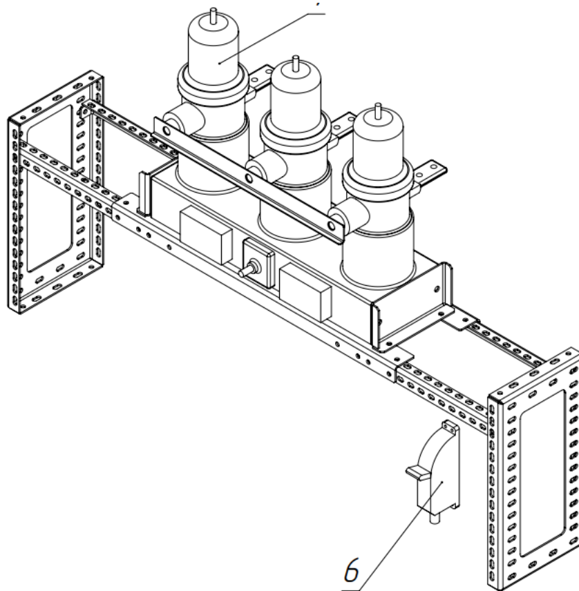
Рис. 14. Соединение рамы адаптации и вакуумного выключателя
